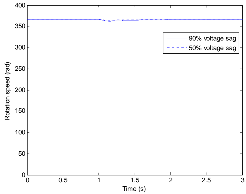
(d) The rotation speed of the rotor (rad/s)
